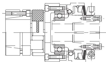
型号DSS/SG/RF，要求设备具备补偿兼容及高抗扭强时，配备无间隙爪形弹性联轴器GAS/SG/CCE。
