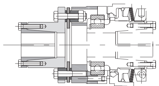
型号DSS/SG/RF，要求设备具备抗扭强度时，配备单件挠性盘式联轴器GTR/S。
