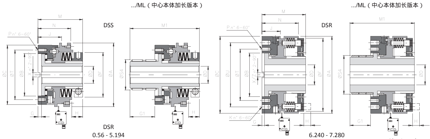
外形尺寸
