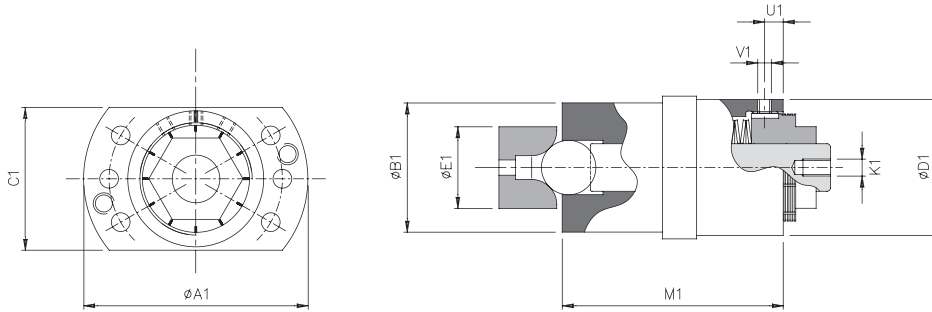
外形尺寸
