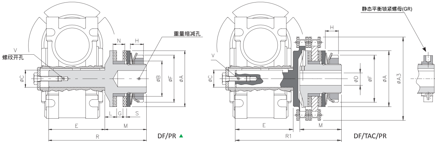
外形尺寸
