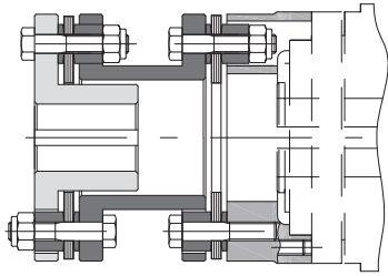
型号 DSS/SG ，当需要配置抗扭强度及具备兼容径向不重合能力时，配备双重挠性扭转力刚性金属盘联轴器 GTR/D 。
