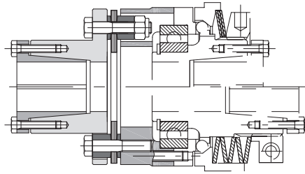
型号 DSS/SG ，需配置抗扭强度功能时，配备单个挠性盘式联轴器 GTR/S 。
